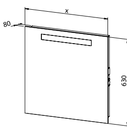
Ogledalo s integriranom rasvjetom, prekidačem i utičnicom 60, 80, 90, 100, 120
