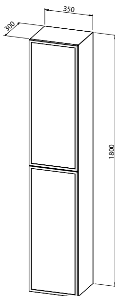
Kolona 35x180 sa staklenim vratima i Al okvirom, 2 vrata, univerzalna - otvaranje na dodir
