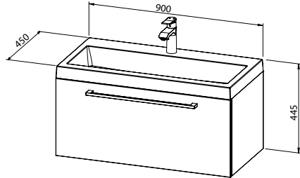
Baza FLORA 90 s umivaonikom, 1 ladica
