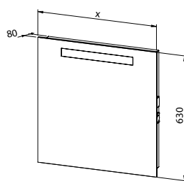
Ogledalo s integriranom rasvjetom, prekidačem i utičnicom 60, 80, 100, 120
