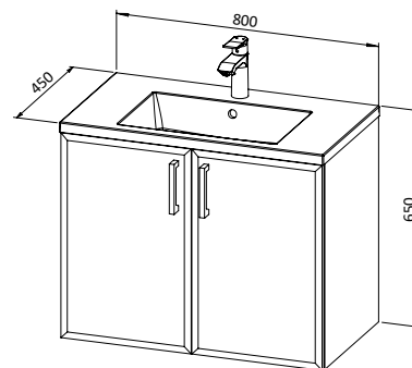
Baza ANA 80 s umivaonikom, 2 vrata
