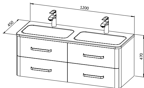
Baza CHARM 120 s umivaonikom, 4 ladice
