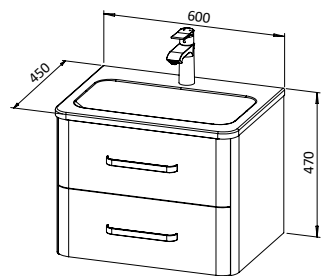
Baza CHARM 60 s umivaonikom, 2 ladice
