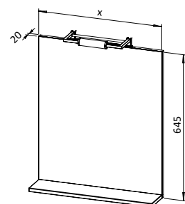
Ogledalo ANA s etažerom, lampicom i prekidačem 55, 80
