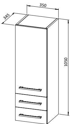
Kolona ASTRA 35x100 , 1 vrata, 2 ladice, viseća, D/L
