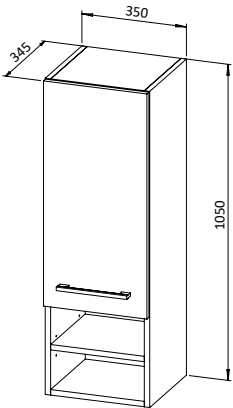
Kolona ASTRA 35x100 , 1 vrata, 1 polica, viseća, D/L
