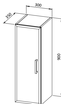
Kolona ANA 30x90 , 1 vrata, univerzalna
