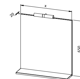
Ogledalo JANA s etažerom, lampicom i prekidačem 40, 50, 60, 80, 100
