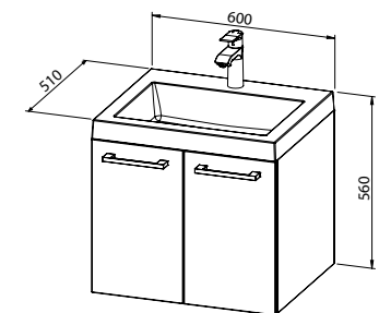
Baza ARWEN 60 s umivaonikom, 2 vrata
