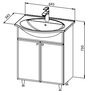
Baza LIDIJA 60 s umivaonikom LUNA 65, 2 vrata
