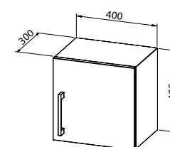
Viseći ormarić ARWEN/FLORA 40 s vratima, univerzalni
