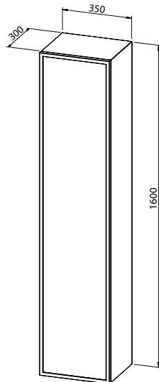
Kolona 35x160 sa staklenim vratima i Al okvirom, 1 vrata, univerzalna - otvaranje na dodir
