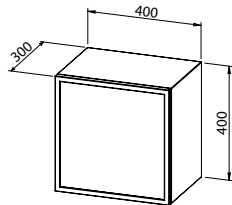
Viseći ormarić 40 sa staklenim vratima i Al okvirom, univerzalni - otvaranje na dodir
