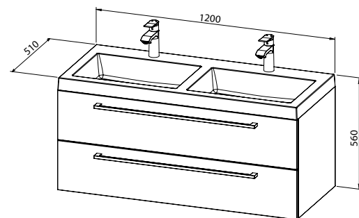
Baza ARWEN 120 s umivaonikom, 2 ladice
