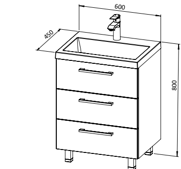
Baza ASTRA 60 s umivaonikom, 3 ladice
