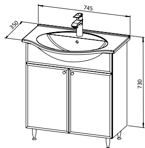
Baza LIDIJA 70 s umivaonikom LUNA 75, 2 vrata
