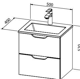
Baza JANA 50 s umivaonikom, 2 ladice
