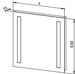
Ogledalo s integriranom rasvjetom, 2 trake 45, 60, 80, 100, 120 - utičnica, senzorski prekidač, LED rasvjeta, grijač protiv magljenja ogledala
