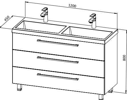
Baza ASTRA 120 s umivaonikom, 3 ladice
