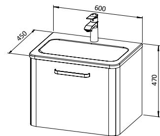
Baza CHARM 60 s umivaonikom, 1 ladica
