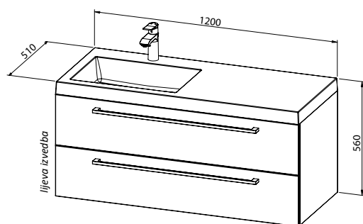
Baza ARWEN 120 s umivaonikom, 2 ladice, L
