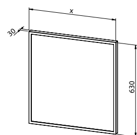
Ogledalo s Al okvirom 40, 60, 80, 100, 120
