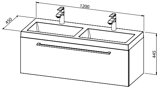
Baza FLORA 120 s umivaonikom, 1 ladica
