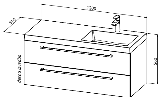
Baza ARWEN 120 s umivaonikom, 2 ladice, D
