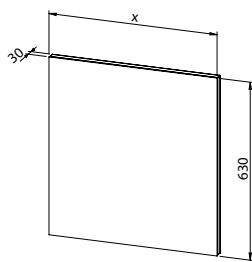
Ogledalo na poledini 40, 60, 80, 90, 100, 120
