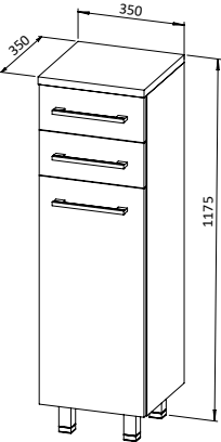
Kolona ASTRA 35x100 , 1 vrata, 2 ladice, D/L opcija: košara za prljavo rublje
