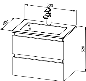
Baza STELLA 60 s umivaonikom, 2 ladice
