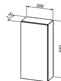
Viseći ormarić 30 s vratima, univerzalni - otvaranje na dodir
