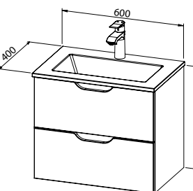
Baza JANA 60 s umivaonikom, 2 ladice
