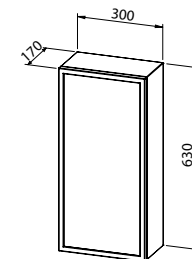
Viseći ormarić 30 sa staklenim vratima i Al okvirom, univerzalni - otvaranje na dodir
