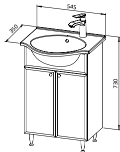
Baza LIDIJA 50 s umivaonikom LUNA 55, 2 vrata
