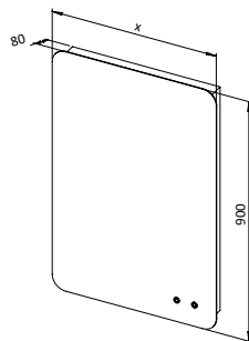
Ogledalo CHARM s pozadinskom rasvjetom 60, 100 - utičnica, 2 senzorska prekidača, LED rasvjeta, grijač protiv magljenja ogledala opcija: LED svjetiljka LINEA
