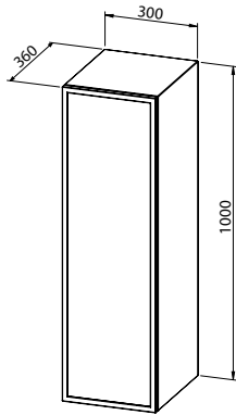
Kolona 30x100 sa staklenim vratima i Al okvirom, 1 vrata, univerzalna - otvaranje na dodir
