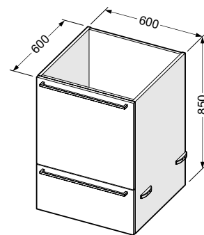
za postavljanje ispod radnog pulta 60x60x84
