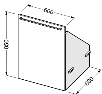
za postavljanje ispod suodpera 60x60x84
