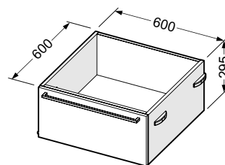
za postavljanje ispod postolja za sušilicu/perilicu 60x60x28,5
