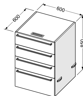
za postavljanje ispod radnog pulta 60x60x84
